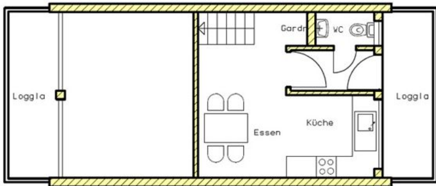
Typ D - 1.Obergeschoss
