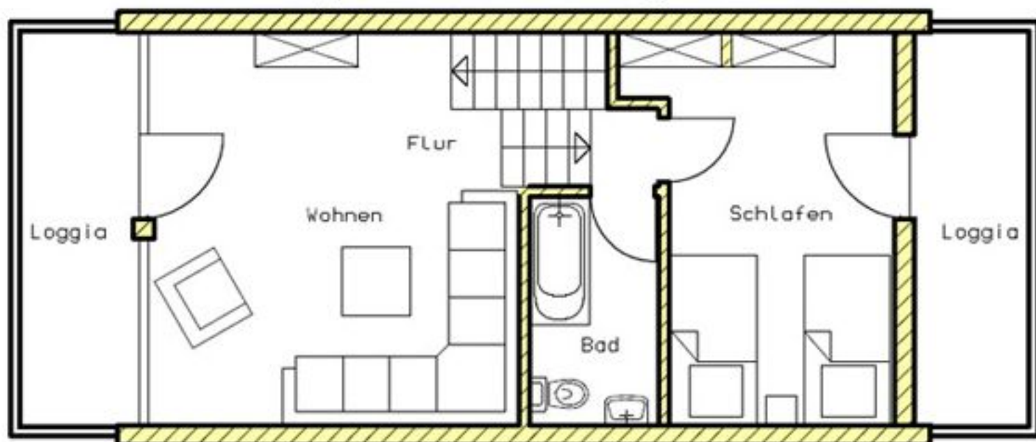
Typ D - 2.Obergeschoss
